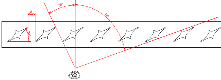
OKASOLAR P 30-08
