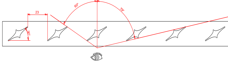
OKASOLAR P 30-23
